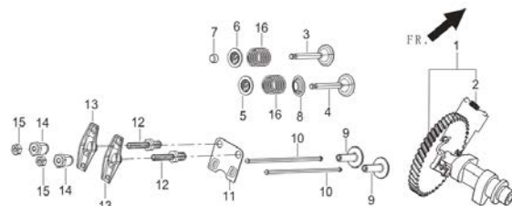
图6：配气机构组件/凸轮轴（E06）
