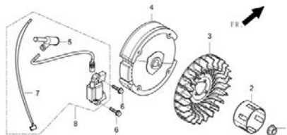
图13：飞轮/叶轮/启动杯/点火线圈（E13）
